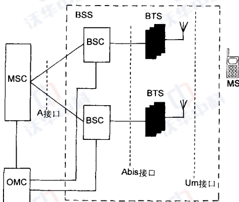
图1 基站设备(BSS)
